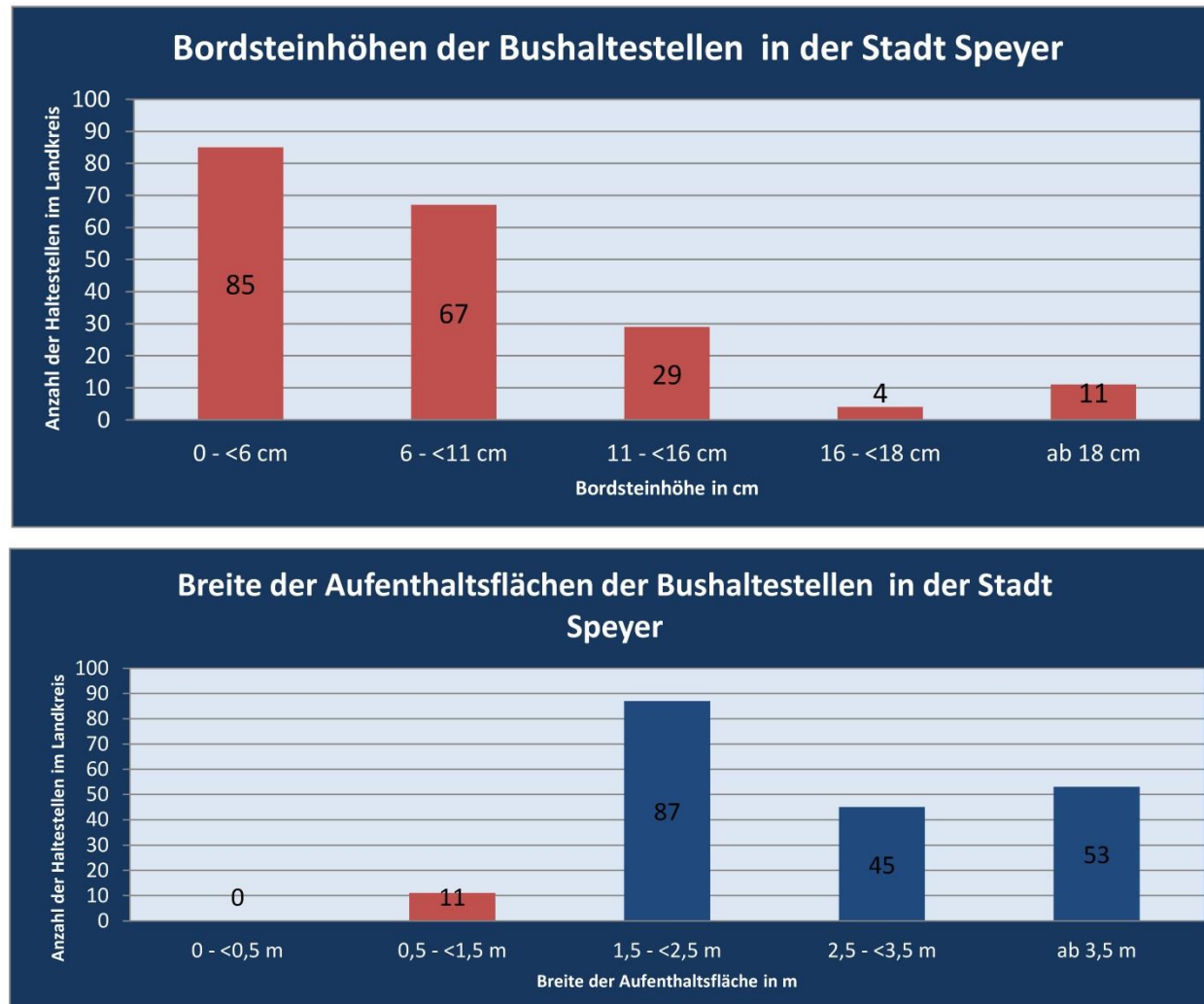
Abbildung 22: Breite der Aufenthaltsflächen und Bordsteinhöhe der Haltestellen in der Stadt Speyer
