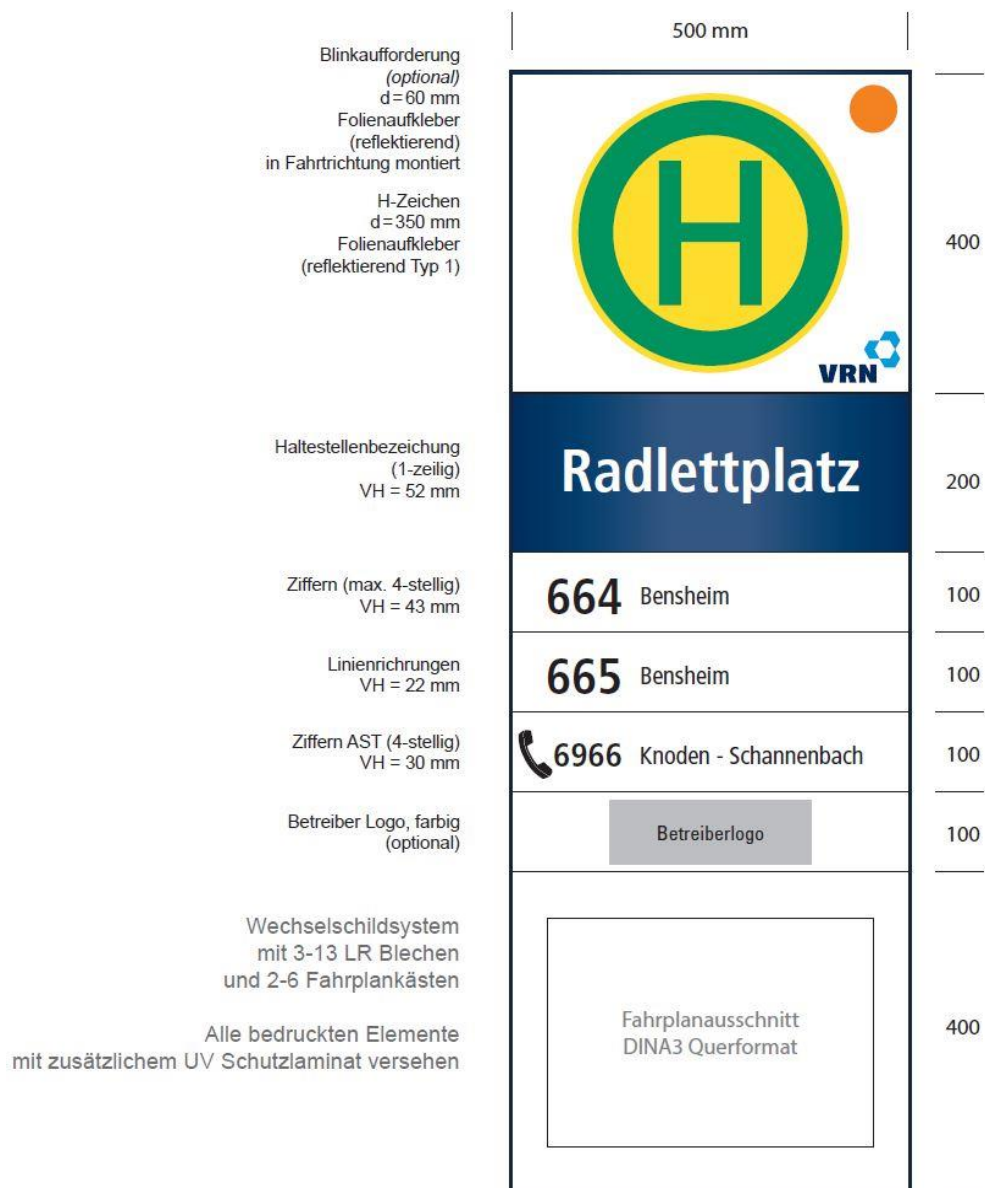
Abbildung 38: Wechselschild mit gewölbter Oberfläche als Stele (höherwertiges System)
