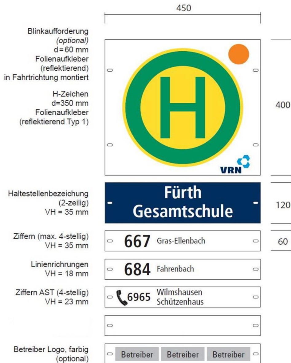
Abbildung 35: Wechselschildsystem (Standard)
